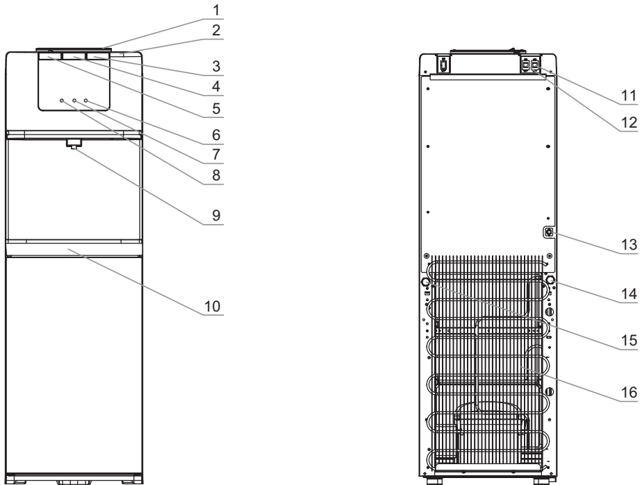
Мал. 1. Схема апарату V8020
