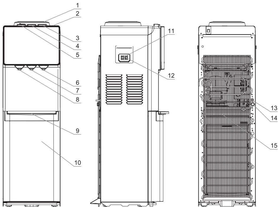
Мал. 1. Схема апарату V400BS
