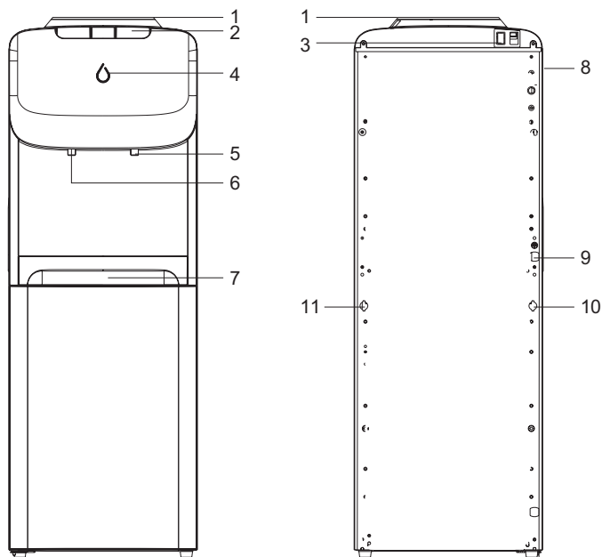
Мал. 1. Схема апарату V170E
