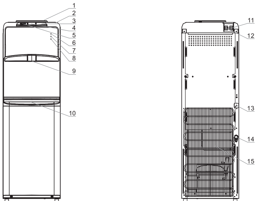
Мал. 1. Схема апарату V100
